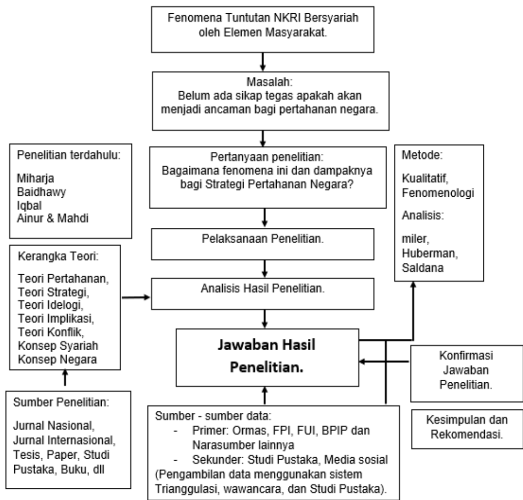
Gambar 2.2 Kerangka Berpikir
