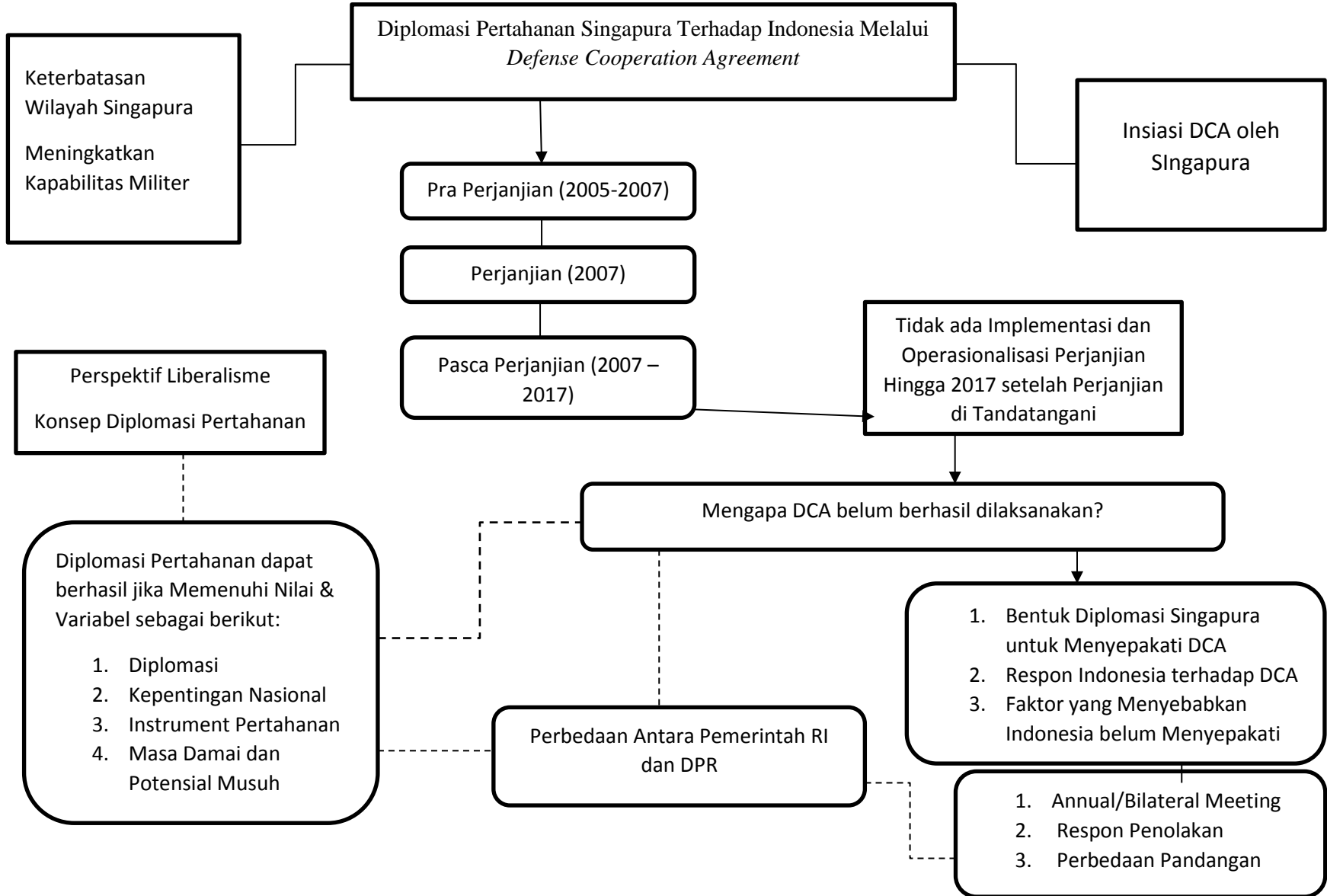
Gambar 2.1 Kerangka Pemikiran
